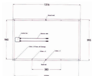
Module dimension
