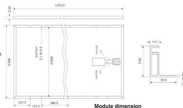
Module dimension
